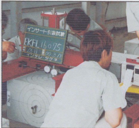
インサート引抜試験風景
